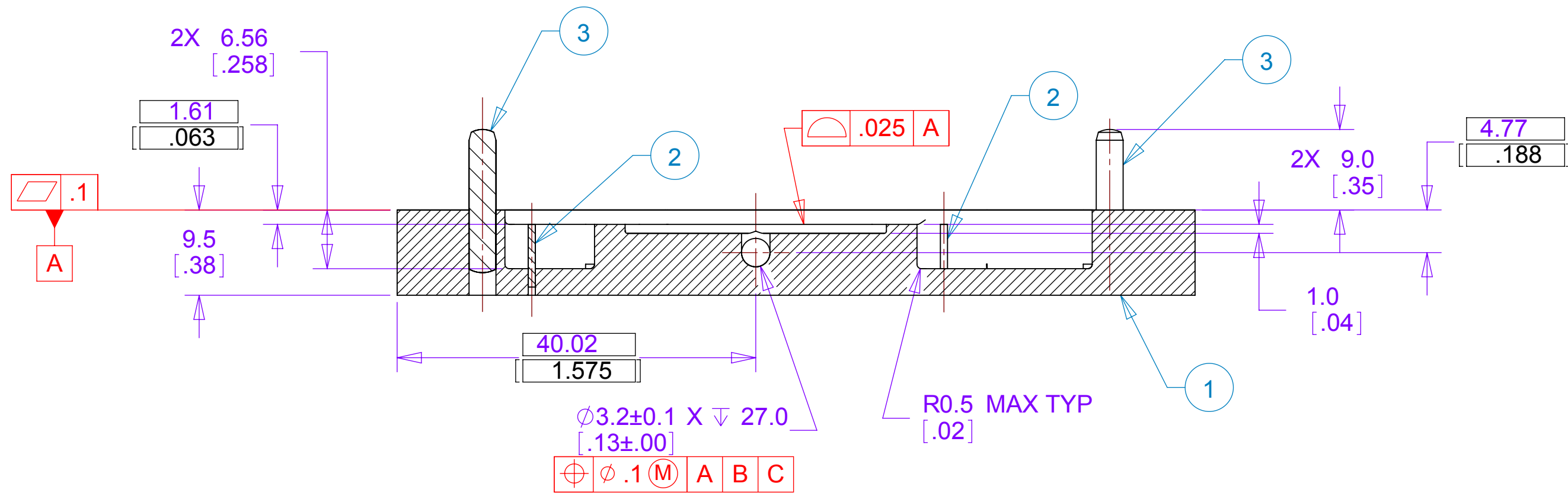
SECTION A-A
